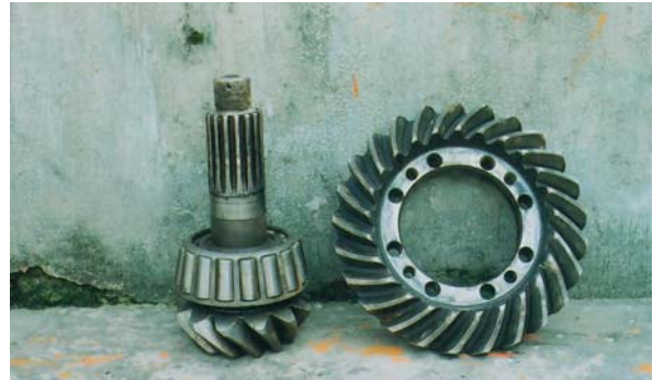
Bánh răng dùng cho Ôtô, tàu thủy, tàu hỏa
